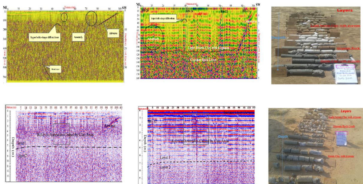
شکل ۵. تفسیر نگاشت‌های راداری با فرکانس ۵۰ و ۲۵۰ MHz مقاطع برداشت GPR با کمک شواهد ژئوتکنیکی گمانه‌ها Fig. 5. Trace (GPR Mapping) interpretation using 50 and 250 MHz GPR sections, supported by geotechnical data from boreholes
